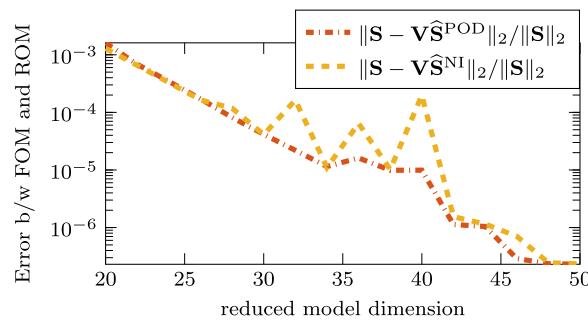
Fig. 11. Batch Chromatography example: Relative errors \|S - \widehat{V}^{\text{POD}}\|_2 / \|S\|_2 and \|S - \widehat{V}^{\text{NI}}\|_2 / \|S\|_2 .
